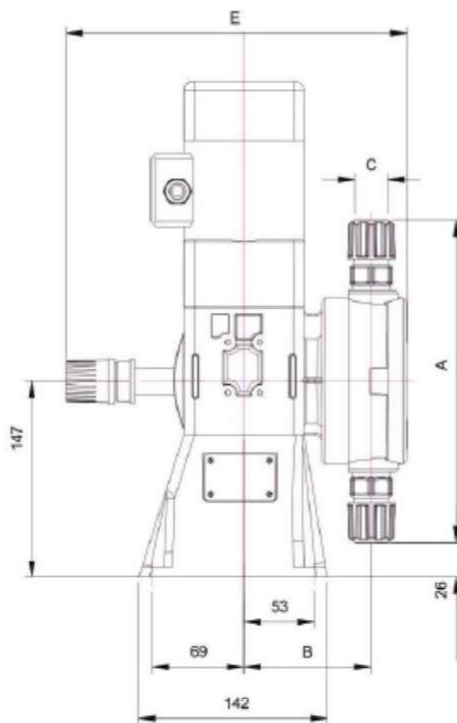
Dati dimensionali - Dimensions
